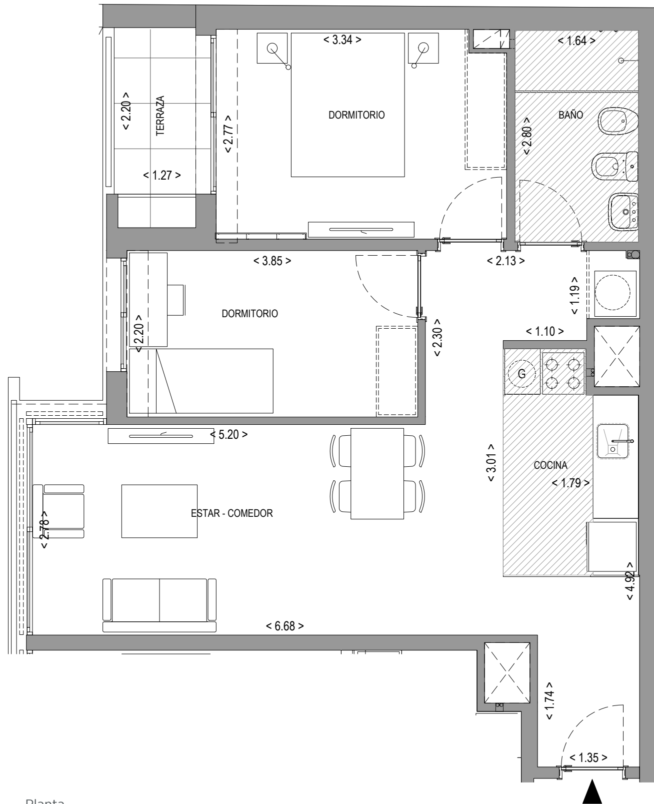
Planta Esc: 1/50
