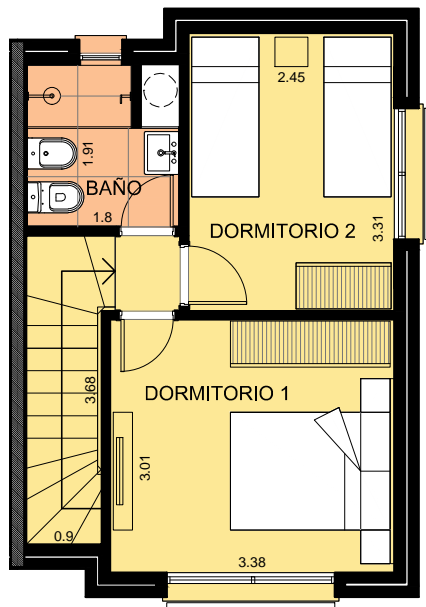
PLANTA ALTA
